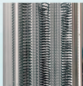
Нихромовые спирали нагревательных элементов
